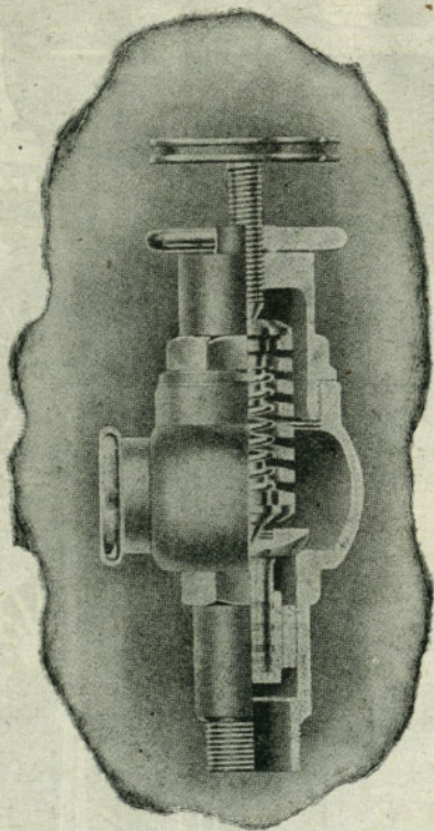
FIG. 24. "E. C. H." RELIEF VALVE.
