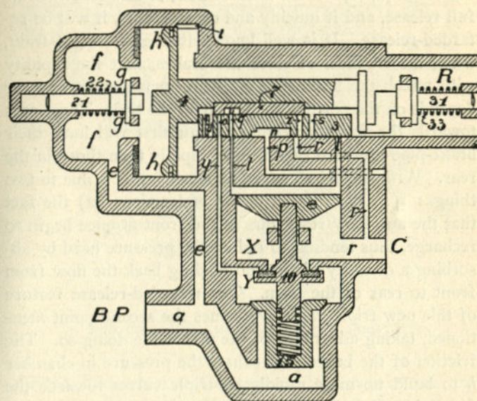
FIG. 329. LAP POSITION
